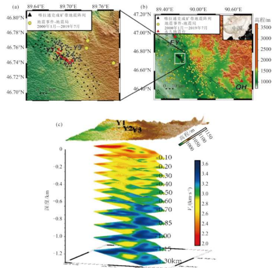
图 10 喀拉通克矿集区地震台阵部署位置及剪切波速度结构 [29]
